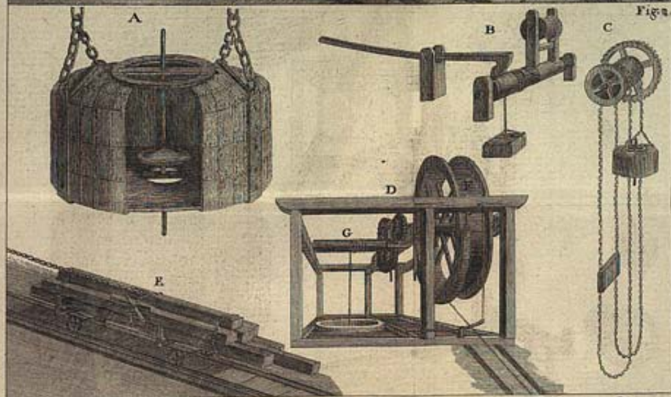
Fig. 1. O Gancho que se solta por si, e qual separa as Cadeas Principaes do outro e Ocaso nas Várias Partes Tambem a Roda Inclinação Com dentes, para impedir o movimento a Cadeas. Fig. 2. A. O Tubo do Gancho. B. O Encontro. C. As Cadeas de Equilibrio. D. O Apparellho para Vellarem as Barras Várias as Almas de Carvão, &c. E. O modo de separarem as Cadeas de qualquer Compimento.
