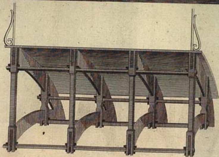
Desenho de 1. Ponte de Ferro. Escala 1. Pollegada até 1o Pé . A Secção mostra as Curvas, e Gatos. Escala 1. Pollegada até 4. Pé
